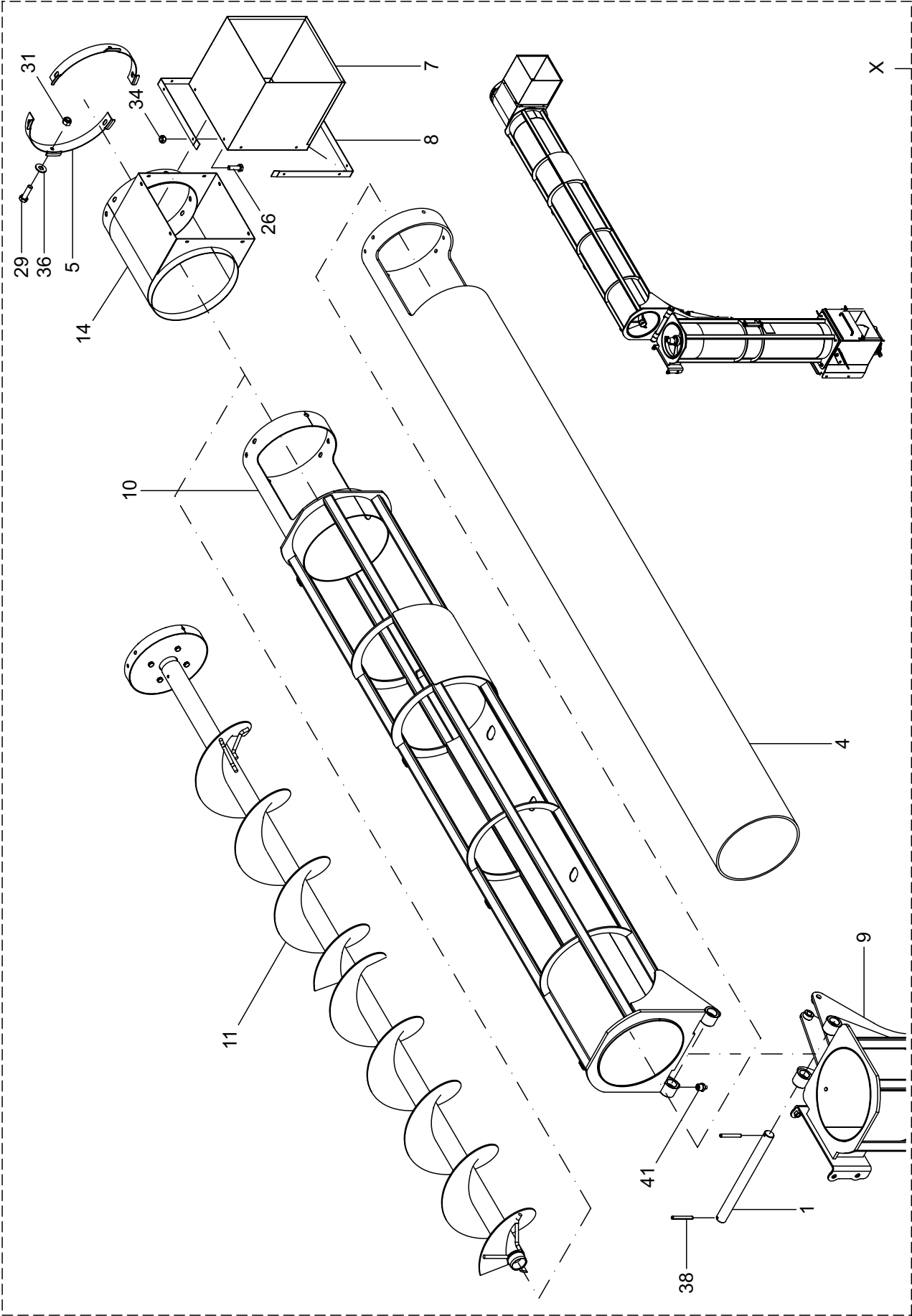
63 - Tubo de descarga multiuso mecánico (opcional) – Tanker Magnu 17.000
