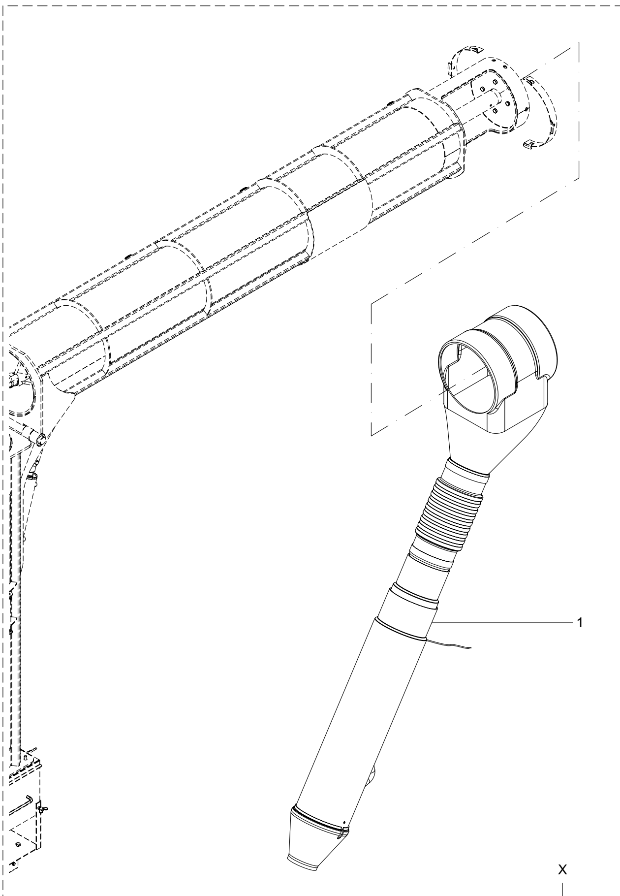
67 - Tubo de descarga multiuso hidráulico (opcional) - Tanker Magnu 17.000 - 20.000 - 25.000
