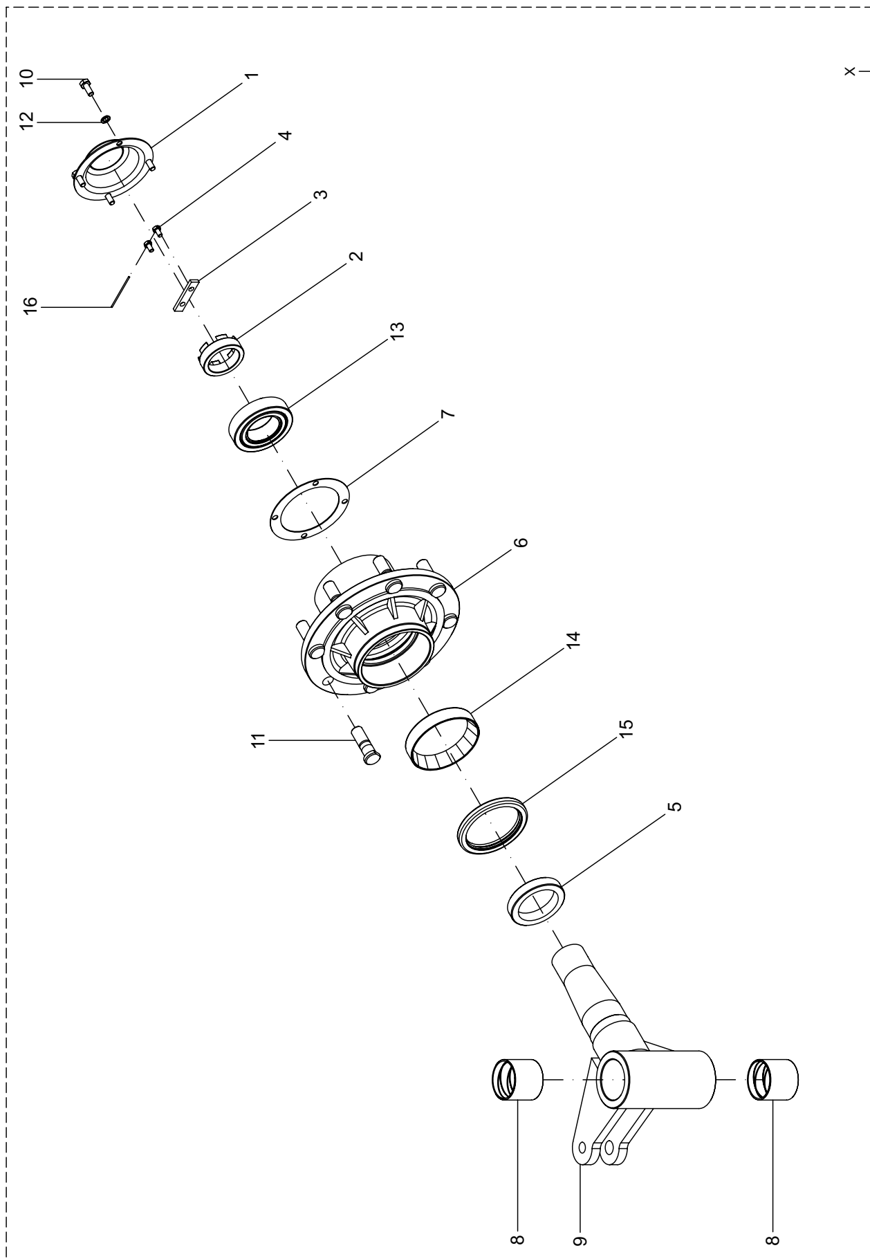
14 - Cubo de rueda izquierdo y derecho – Tanker Magnu 17.000
